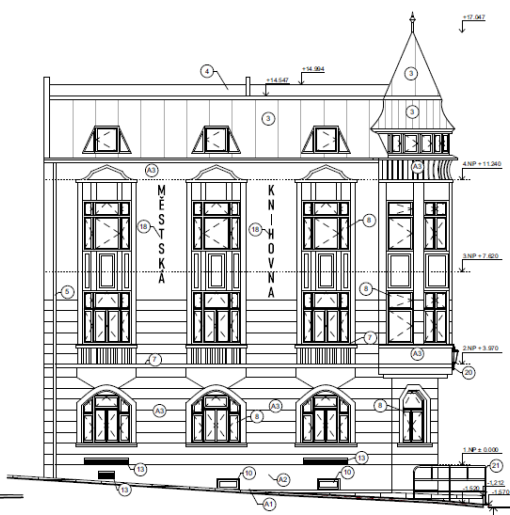
POHLED SEVEROZÁPADNÍ
